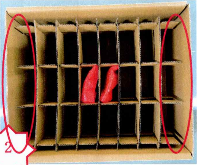
图二，每小格放 1 个 MP02047 组件，每层共计 18 个组件，共计 1 层
